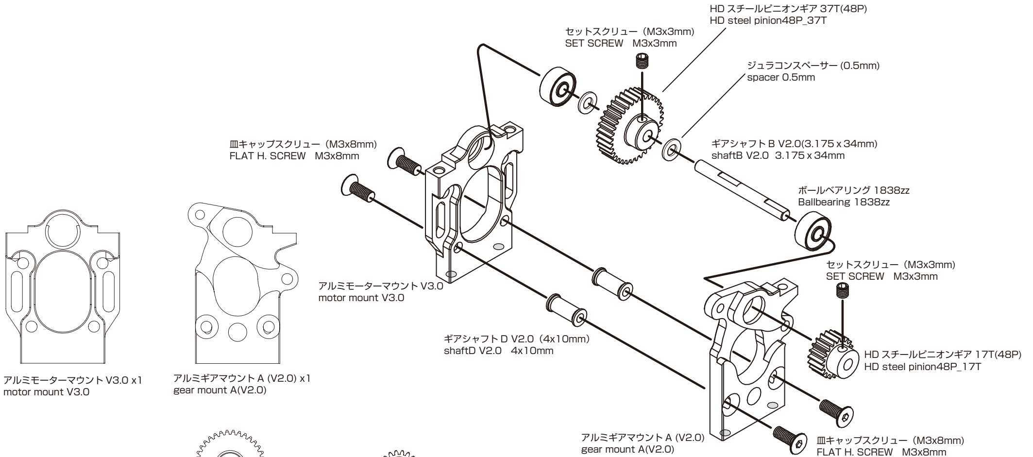
ギアシャフト B V2.0(3.175 x 34mm) shaftB V2.0 3.175 x 34mm
