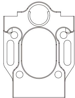
アルミモーターマウント V3.0 x1 motor mount V3.0
